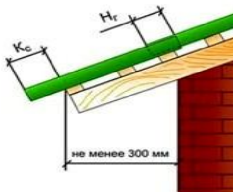
Рис. 1 Карниз кровли
